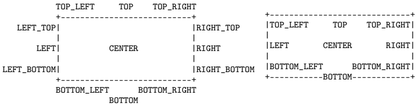
Рис. 10.11. Константы для обозначения положения метки
