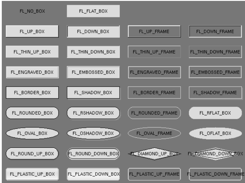
Рис. 10.8. Типы оформления виджетов FLTK 36
