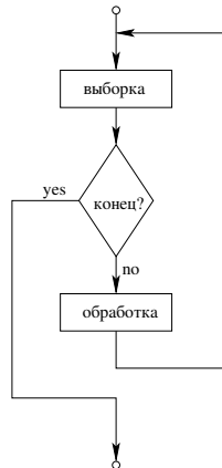
Рис. 4.4. Блок-схема цикла с побочным эффектом в условии
