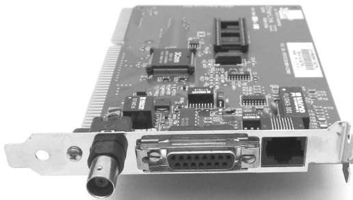
Рис. 6.3. Сетевая карта 3c509 (ЗСОМ) с разъёмами для подключения коаксиального кабеля (слева), внешнего адаптера (в центре) и кабеля витой пары (справа).
