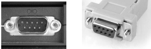
Рис. 5.7. Порт RS-232: разъём (слева 32 ) и штекер (справа)
