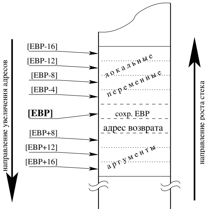
Рис. 3.5. Структура стекового фрейма
