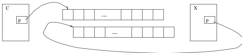
Рис. 2.2. Схема структуры данных после применения конструктора копирования
