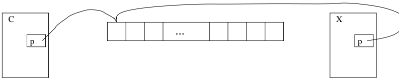
Рис. 2.1. Схема структуры данных после побитового копирования объекта
